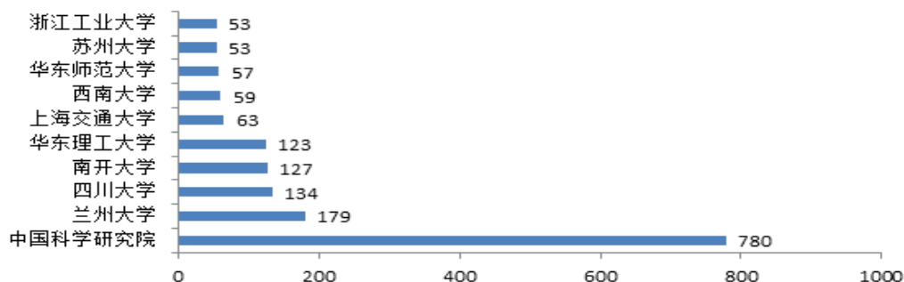
图 4 中国相关施引文献涉及机构 (TOP10)
