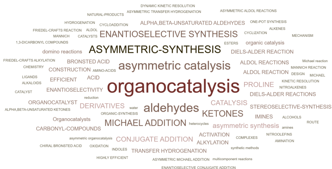
图 5 全球施引文献关键词词云图
