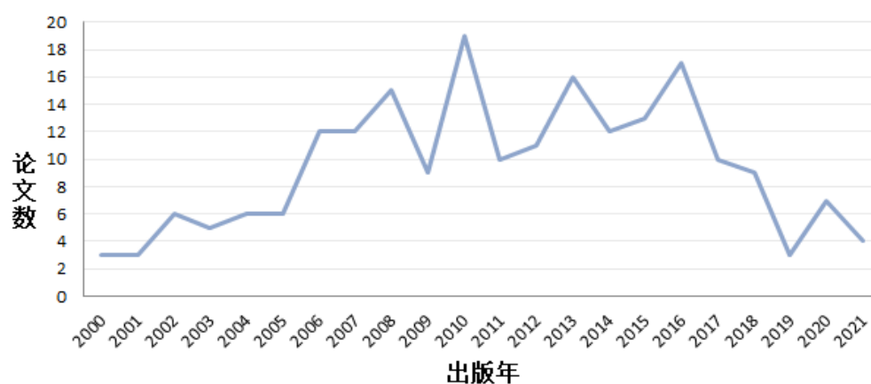
图 1 诺贝尔化学奖获得者相关主题论文年度分布
